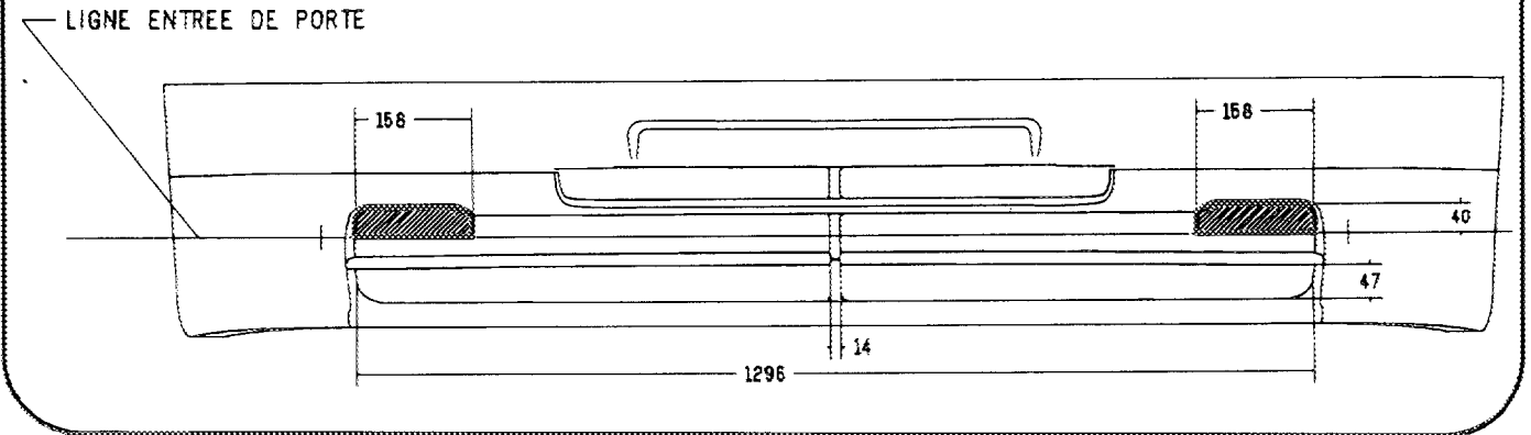
A1) Ouverture dans le capot moteur Opening in engine bonnet
